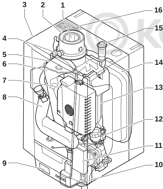
Рис.1 PMC-S 24 – 34
