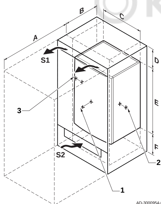
Рис.3 Зона установки
