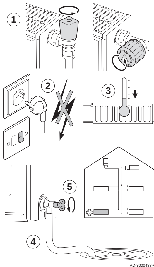
Рис.96 Слив системы
