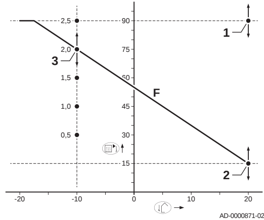
Рис.66 Внутренний график нагрева
