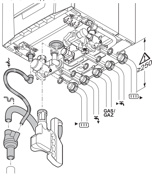
Рис.20 Подключить
