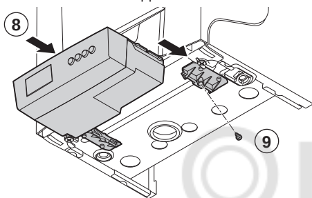
Рис.25 Монтаж соединительного блока
