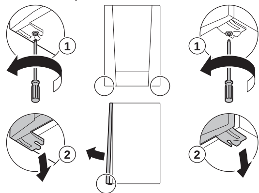
Рис.67 Открытие котла
