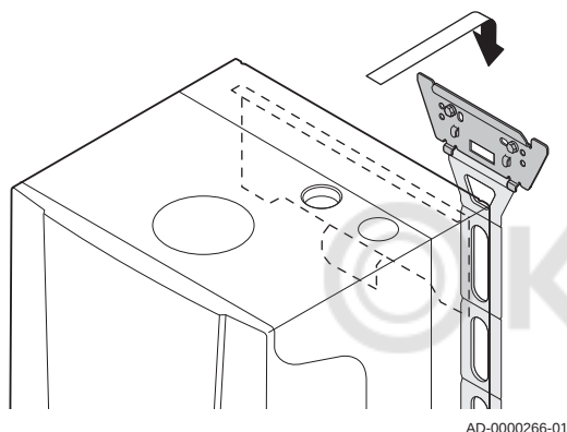
Рис.19 Установка котла
