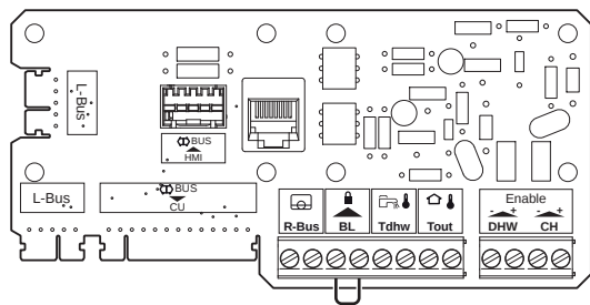
Рис.26 Стандартная управляющая электронная плата (CB-06)
