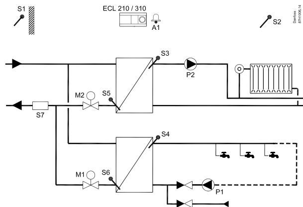
Стандартная схема A266.1:
