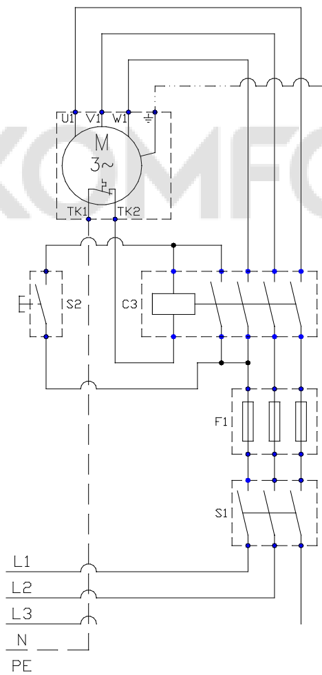
Tri fazni motor termično varovan s termo kontaktom (TKO)
