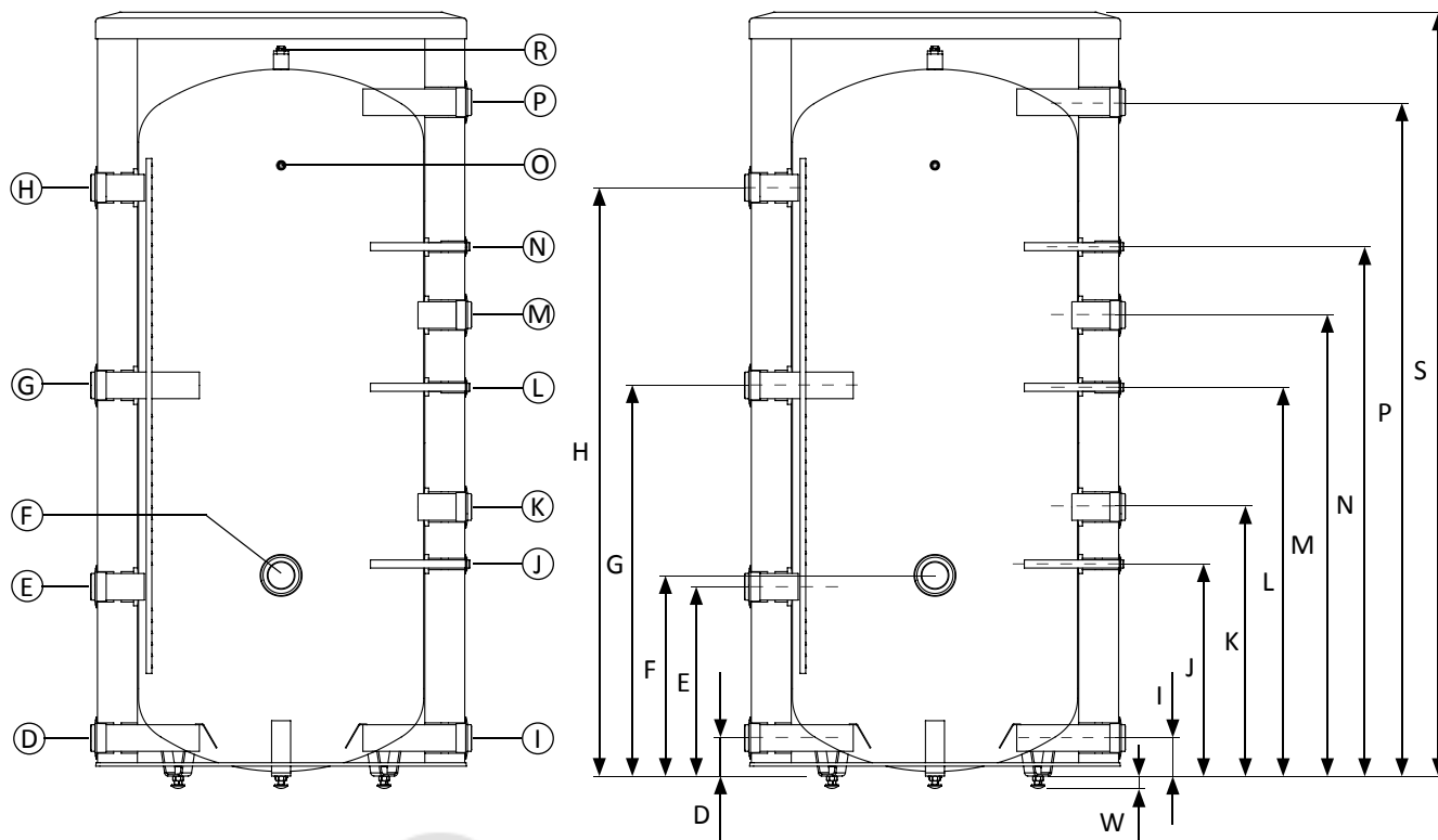
Рис. 17. Размеры теплоаккумулятора BU-750 - 1000.8 R
