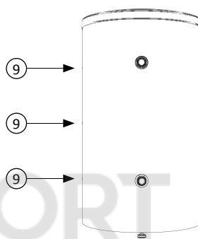
Рис. 6 Теплоаккумулятор BU-200.8 R (вид сбоку)
