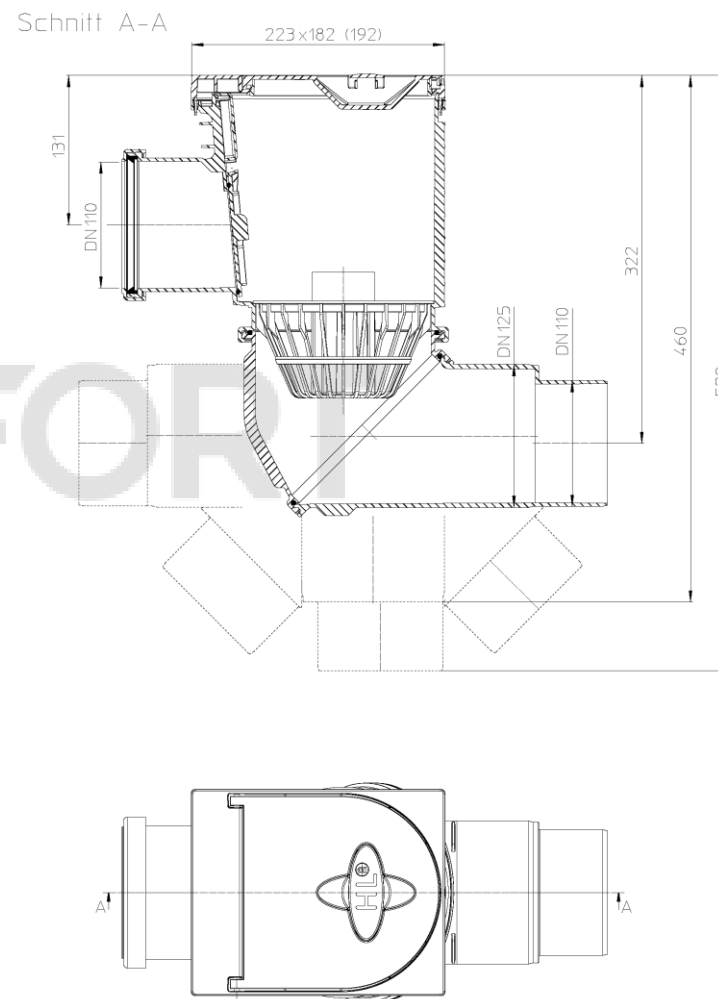
Рис. 1. Дождеприемник HL600NHO.
