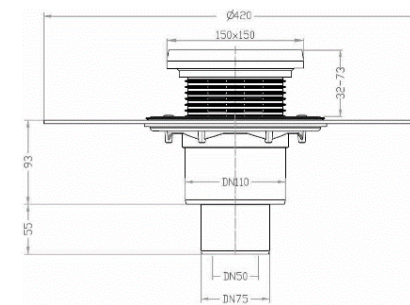
Трап HL310NHPrG
