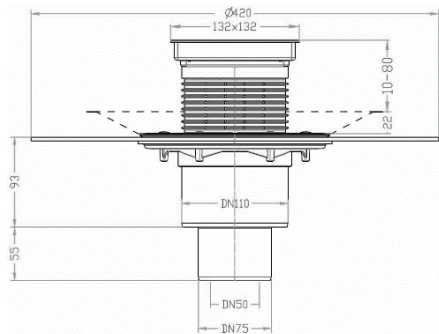
Трап HL310NH-3020
