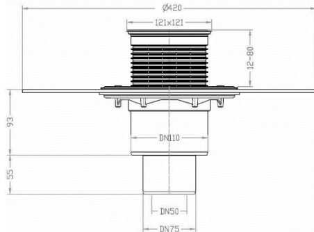
Трап HL310NH-3000
