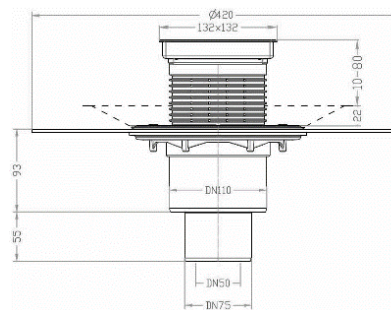
Трап HL310NHPr-3020
