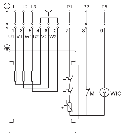
Билдиргичтери менен жасалган Термоөчүргүч, резистор RT1000, нымдуулук релеси жана майдагы сууну билдиргич
