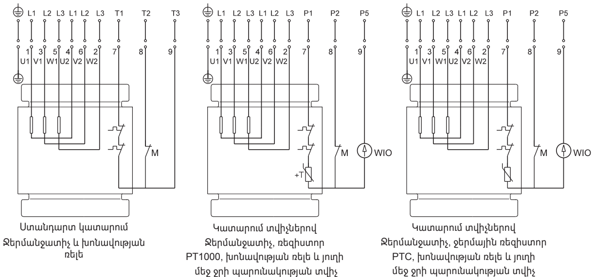
Նկար 7 10-ջիղանի մալուխի համար էլեկտրական միացումների սխեմաներ, միացում, աստղ-եռանկյունի (Y/D)
