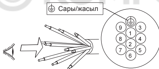
8-сур. 10-тармақты кабельге арналған электр жалғаулар схемасы, «жұлдызша» жалғауы (Y)
