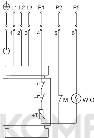
Датчиктармен орындалу Термоажыратқыш, PT1000 резисторы, ылғалдылық релесі және майдағы су датчигі
