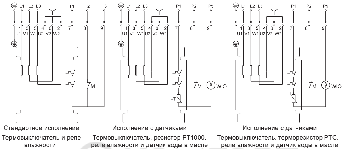
Рис. 8 Схема электрических соединений для 10-жильного кабеля, соединение «звезда» (Y)
