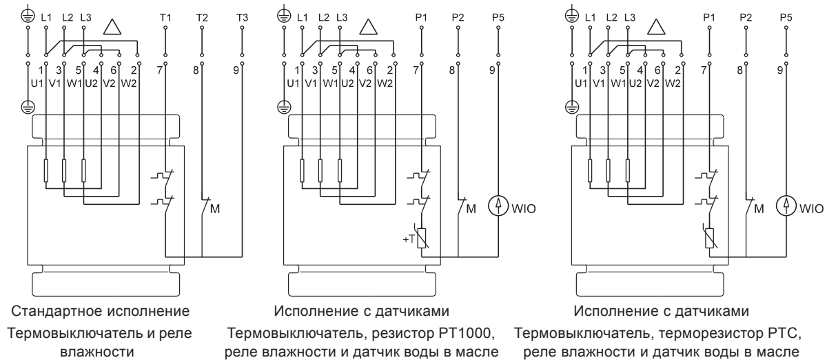
Рис. 9 Схема электрических соединений для 10-жильного кабеля, соединение «треугольник» (D)
