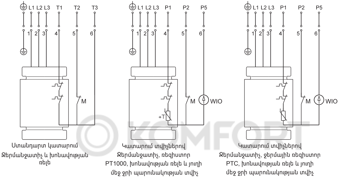
Նկար 6 7-ջիղանի մալուխի համար էլեկտրական միացումների սխեմաներ, ուղղակի մեկնարկ
