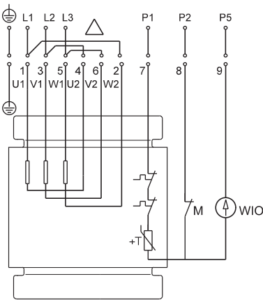
Билдиргичтери менен жасалган Термоөчүргүч, резистор RT1000, нымдуулук релеси жана майдагы сууну билдиргич
