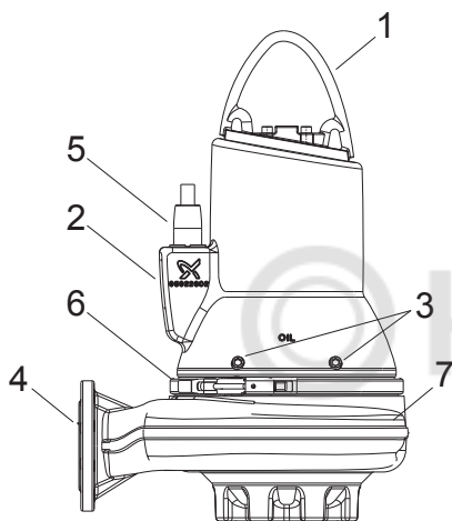
Сүр. 1 Соркысма SL1
