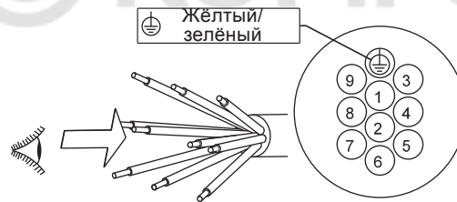
Рис. 8 Схема электрических соединений для 10-жильного кабеля, соединение «звезда» (Y)
