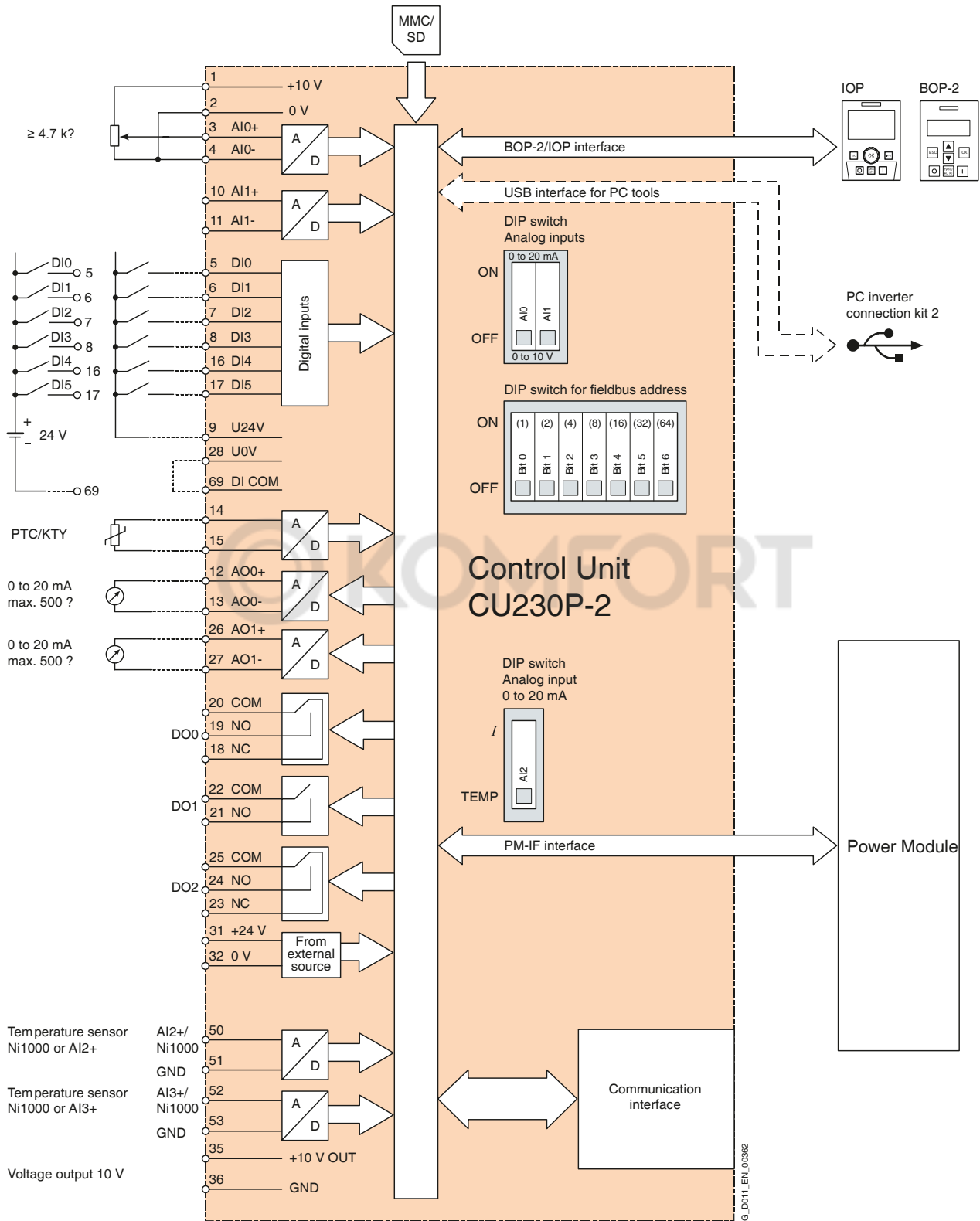
Диаграмма соединений управляющего модуля CU230P-2 ВТ.
