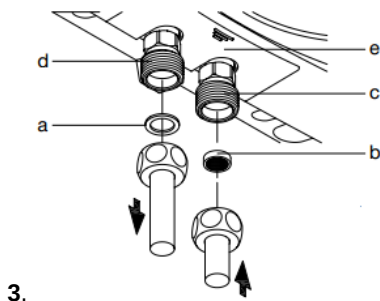
Малюнок 3. Встановлення над раковиною
