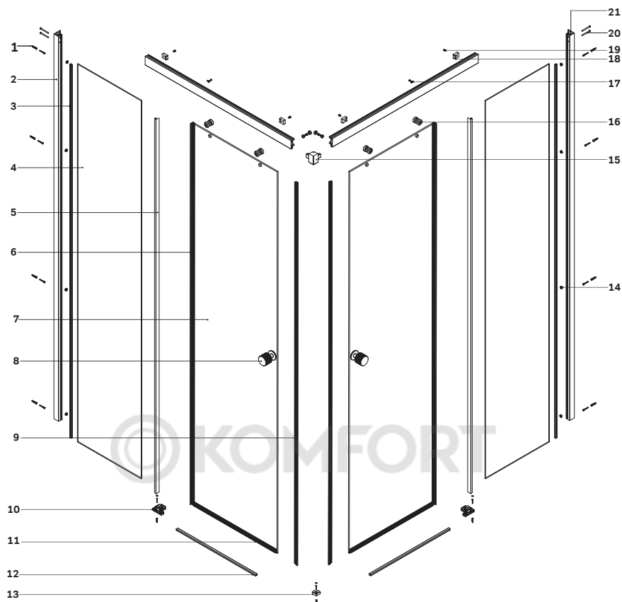
Gehäuse kon igation / Enclosure con igation / Комплектация ограждения 90x90, 100x80, 120x80, 120x90
