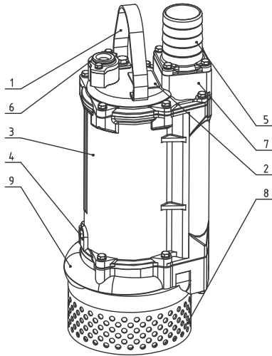
Рис. 2 Насос DWK
