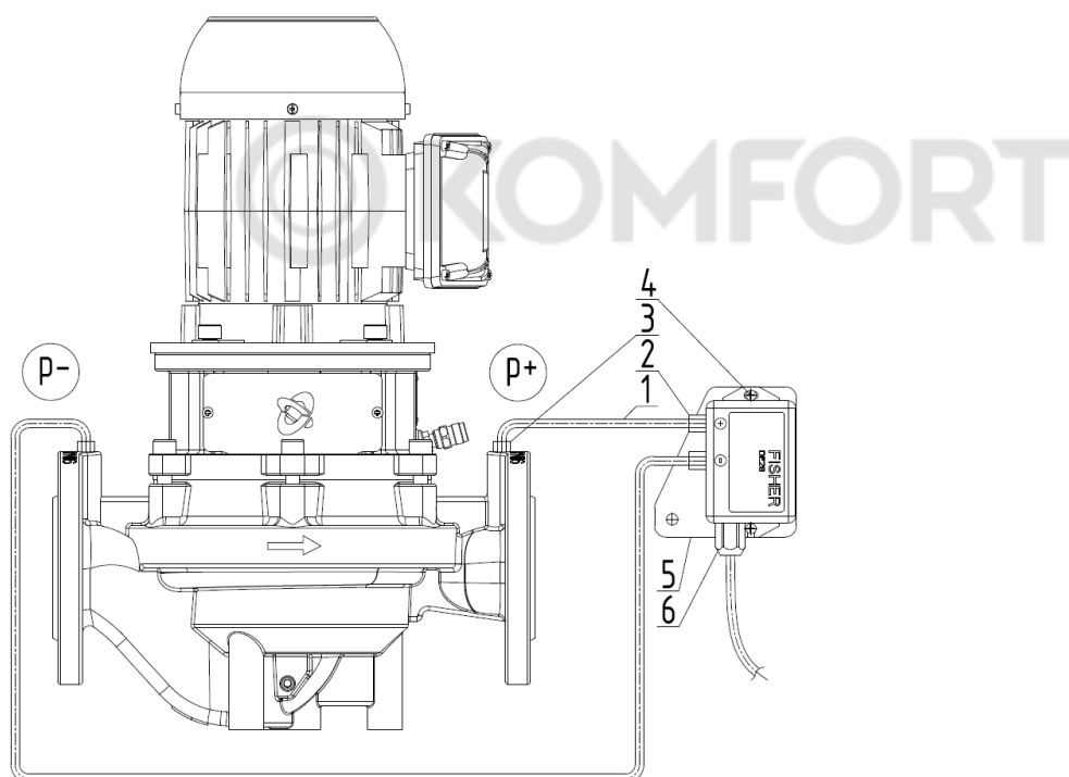
Abbildung 1: Schematische Darstellung der Montage des Druckmessers DE28
