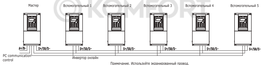
Рис. 19 Контурная схема
