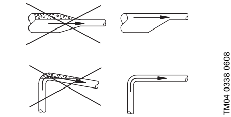
Рис. 2 Трубная обвязка
