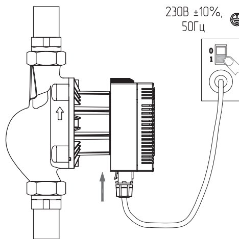
Рис. 36 Электроподключение насоса
