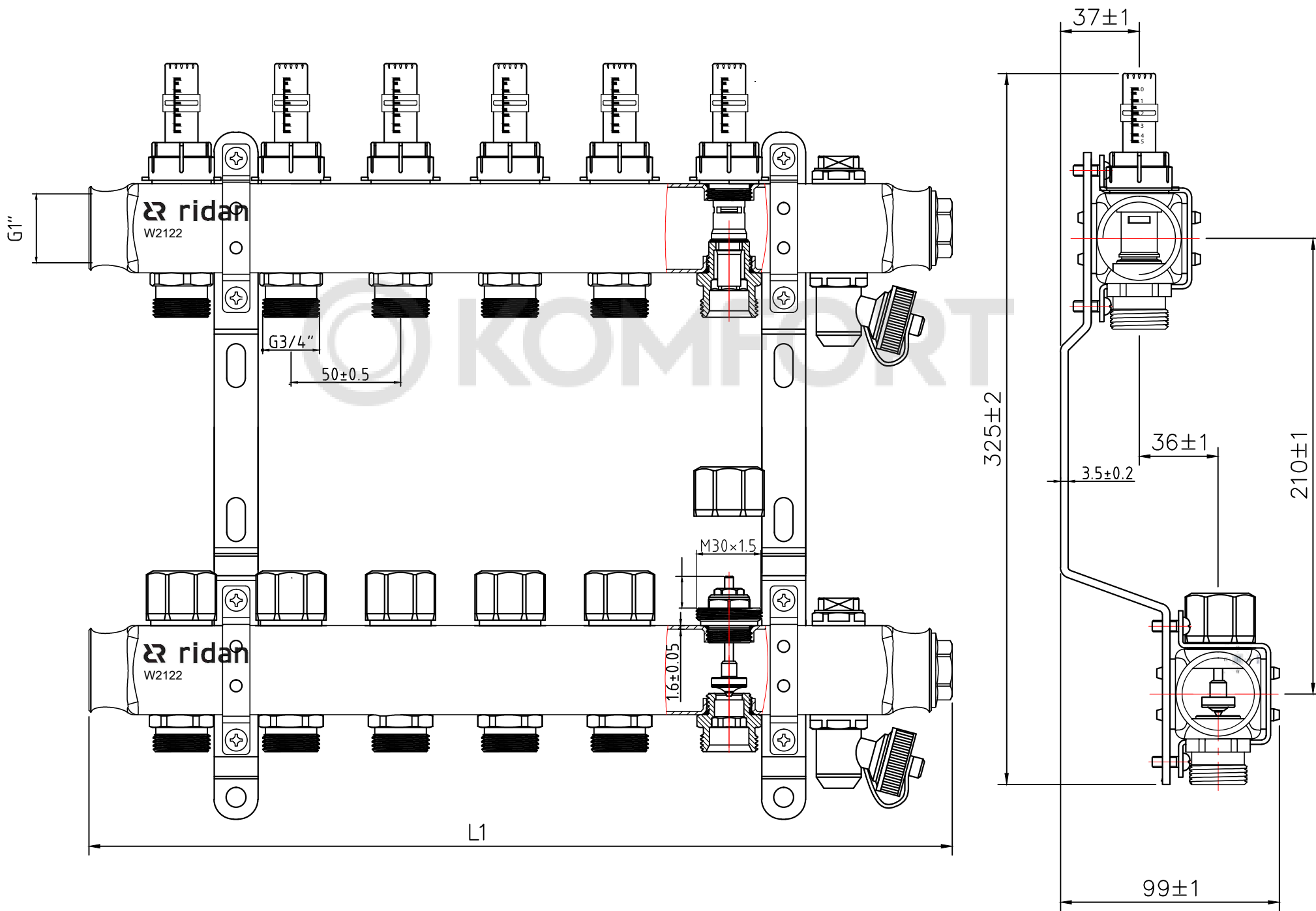
Габаритные размеры
