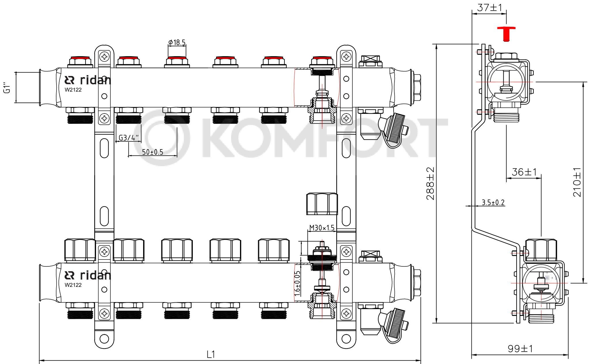
Габаритные размеры
