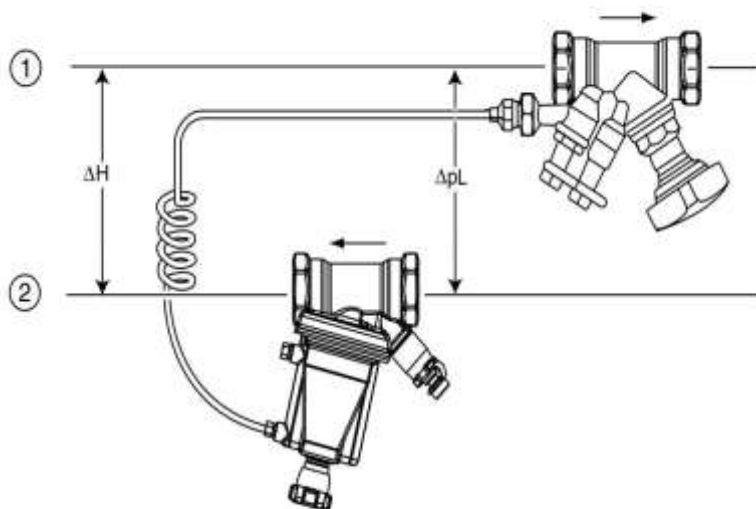
Схема установки
