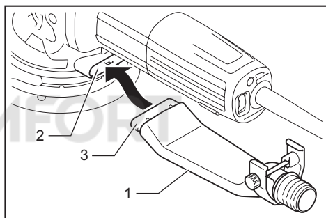
1. Пылесборный патрубок 2. Выходное пылесборное отверстие 3. Раструб
