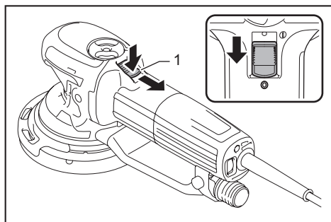
1. Ползунковый переключатель
