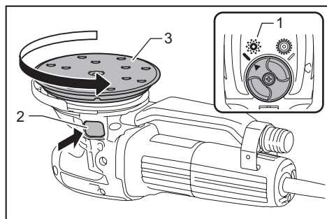
1. Режим эксцентриковой шлифмашины с принудительным вращением 2. Кнопка замка вала 3. Подушка
