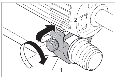
1. Держатель 2. Болт
