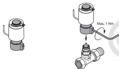
Привод TWA-A NC
