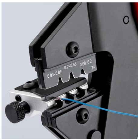
97 43 200 с матрицей опрессовочной 97 49 24 и с устройством поддержки позиционирования 97 49 93 для штекера типа D-Sub
