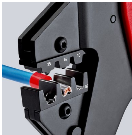
97 43 200 с матрицей 97 49 09 для контактных гильз
