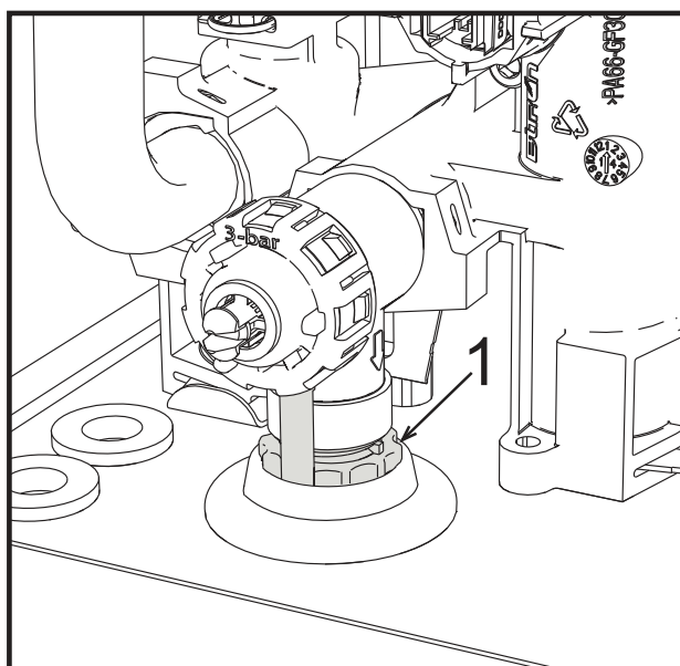
рис. 10- Предохранительный клапан со сливным краном
