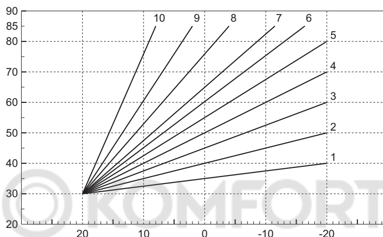
рис. 25- Компенсационные кривые
