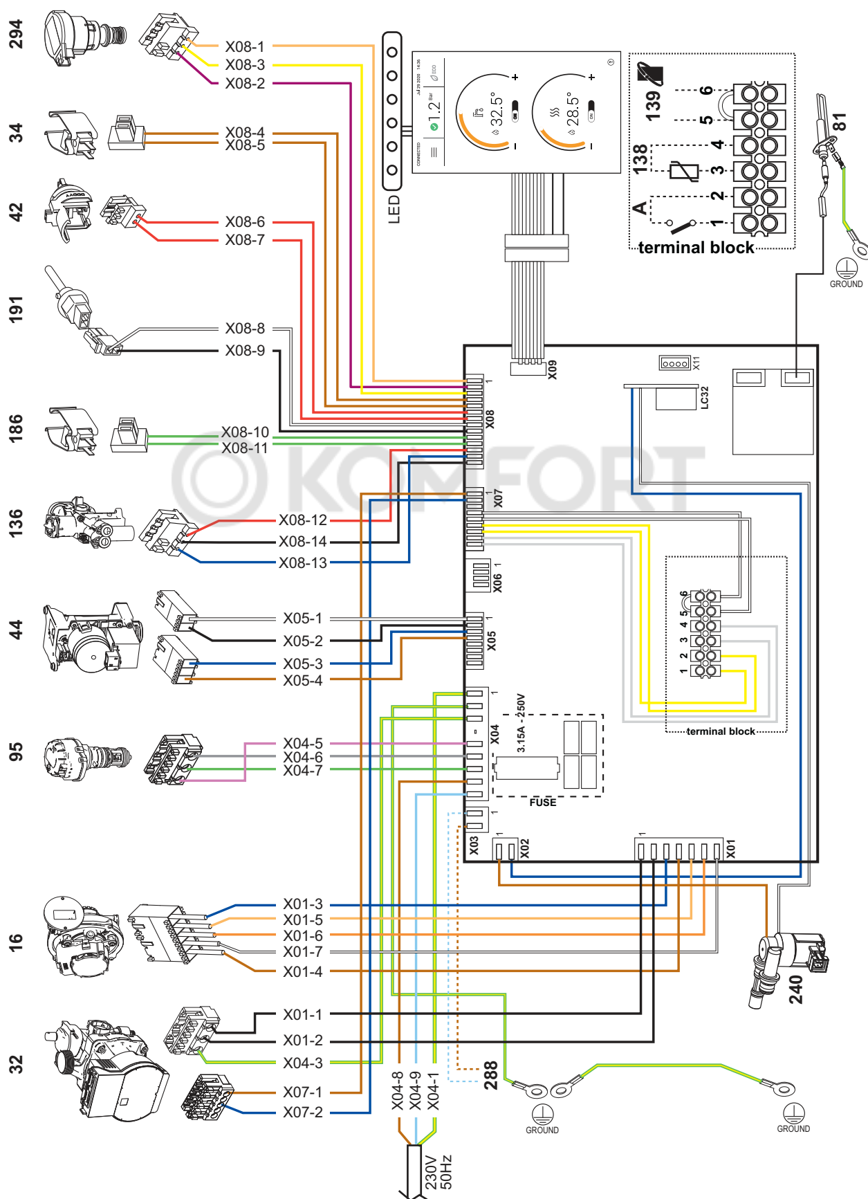
рис. 46- Электрическая схема
