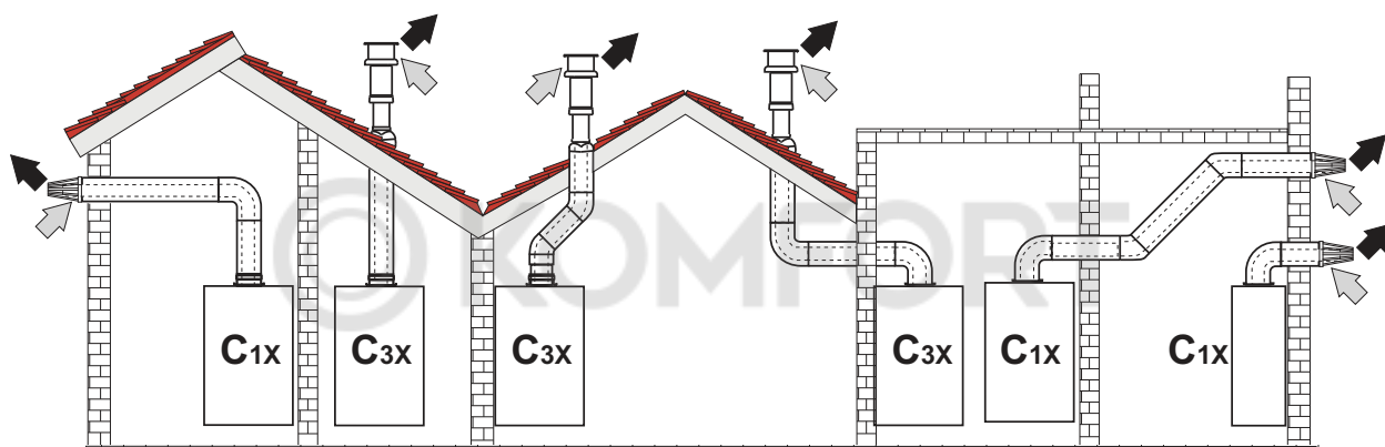
рис. 14- Примеры подсоединения с помощью коаксиальных труб (⇐ = Воздух/ ⇨ = Дымовые газы)
