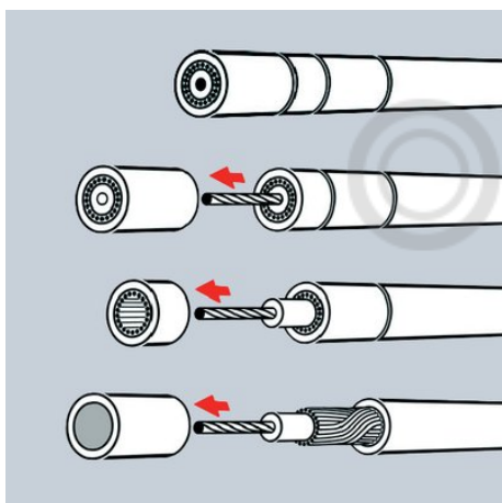
Трехступенчатое удаление изоляции с коаксиального кабеля
