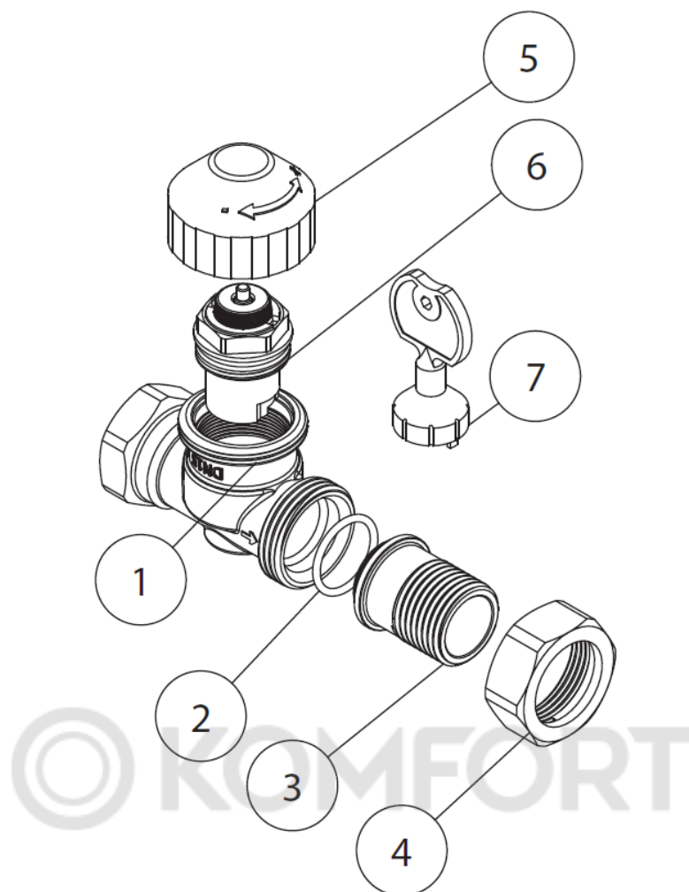
Рисунок - Устройство клапанов терморегулирующих типа TR-N
