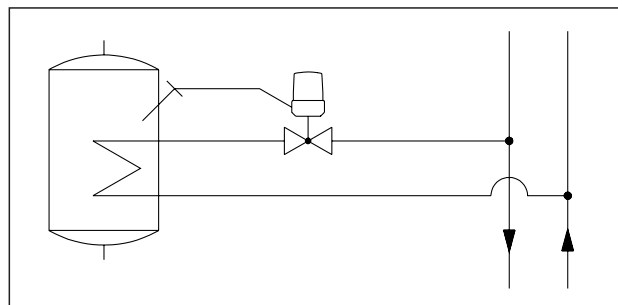
Бойлер-накопитель
