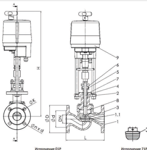
Исполнение 01P
