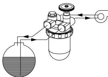
Фильтр „Oilpur” для двухтрубной системы
