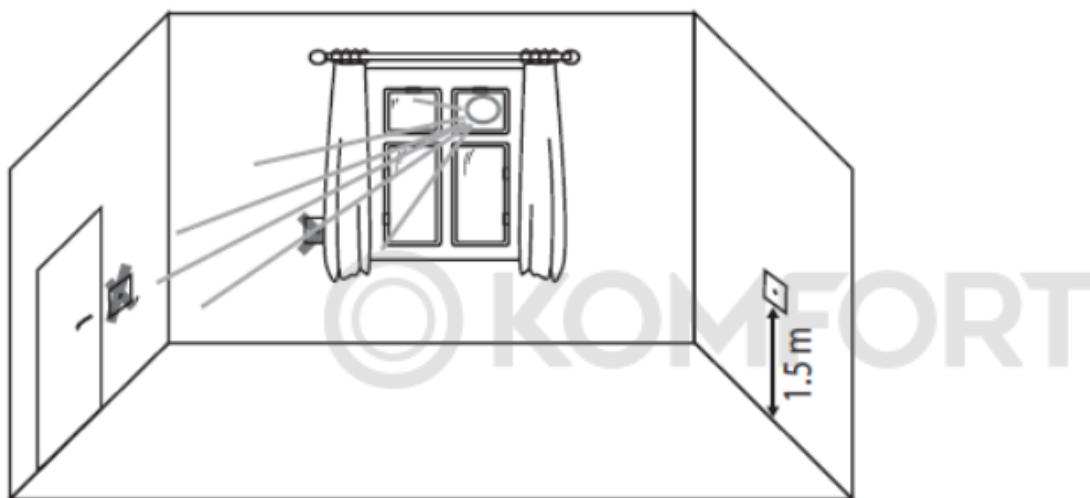
Рис. 5. Рекомендуемые и запрещённые к установке зоны расположения терморегулятора EStemp™ Next Plus.
