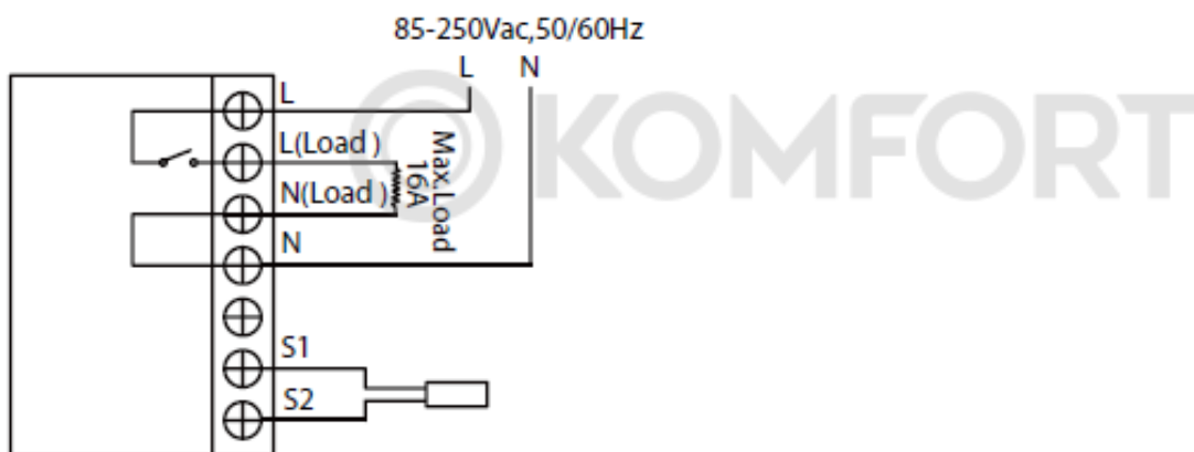
Рис. 7. Монтажная электросхема EStemp™ Next Plus.
