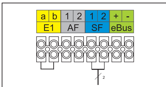
Рисунок. Соединение датчика бойлера
