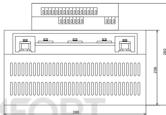
Вид снизу
