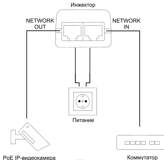
Рисунок 2 – схема подключения
