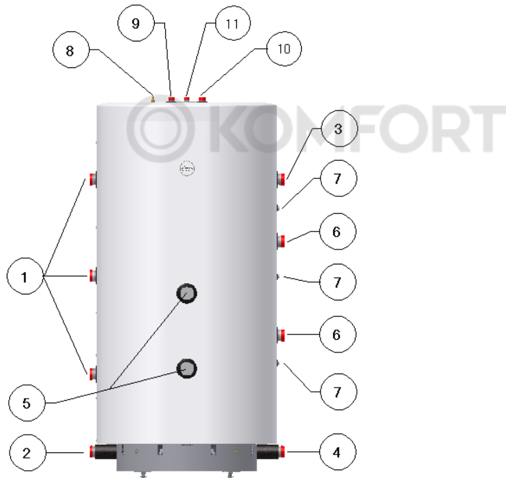
BUZ – 750/200.90 R, BUZ – 1000/200.90 R – вид спереди
