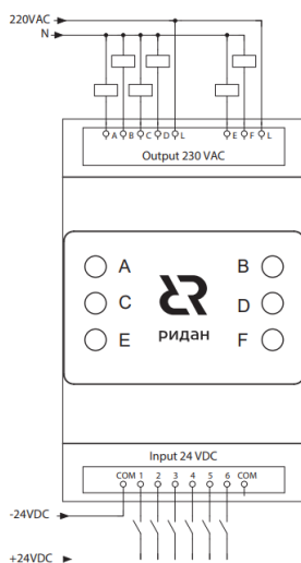
Рис. 2 Схема подключения модуля P-PM
