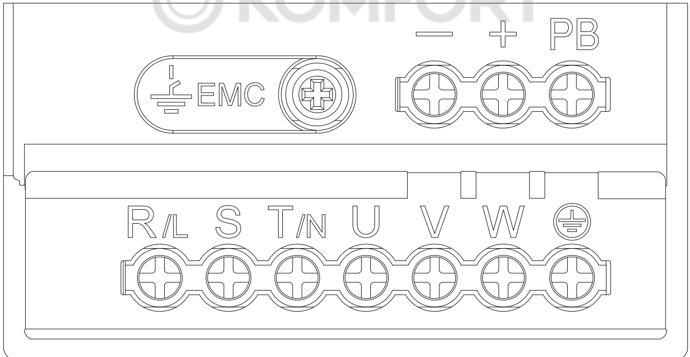
Рисунок 3.1-2 Расположение клемм
