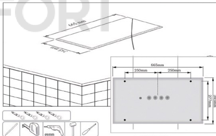
Вид снизу
