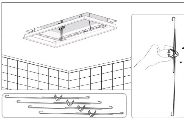
Вид снизу
